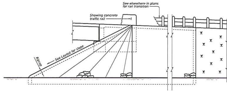
ELEVATION
